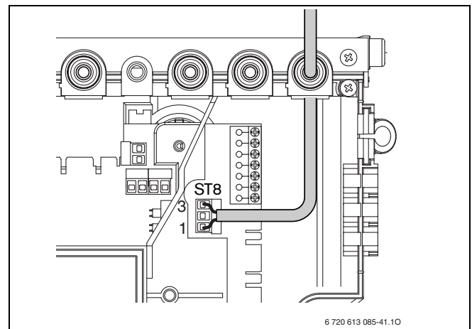
23. ábra Melegvítároló termosztát-csatlakozása
