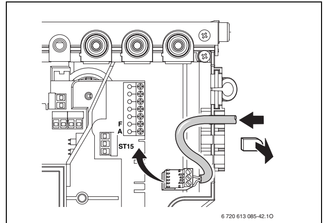
22. ábra A melegvítároló hőmérséklet-érzékelőjének (NTC) csatlakozása
